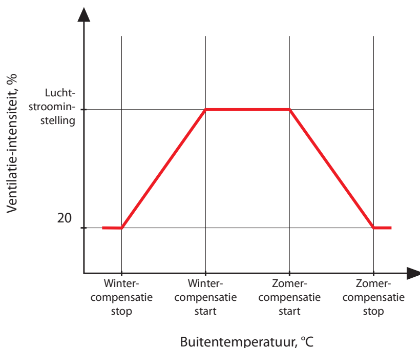
Fig. 1. OCV-functiebediening
