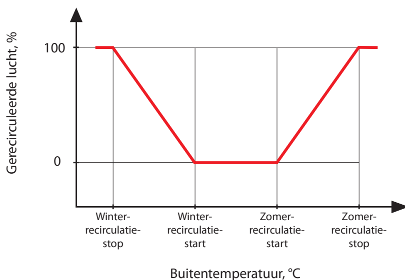
Fig. 2. REC-functiebediening
