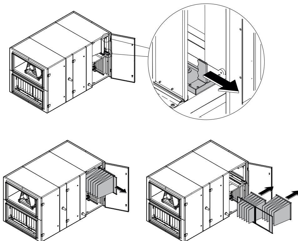
Fig. 3. Filterklemminrichting
