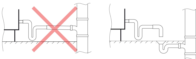
Fig. 23. Aansluiting van de condensaatafvoer op de riolering
