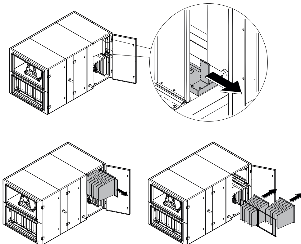
Fig. 44. Filterkleminrichting
