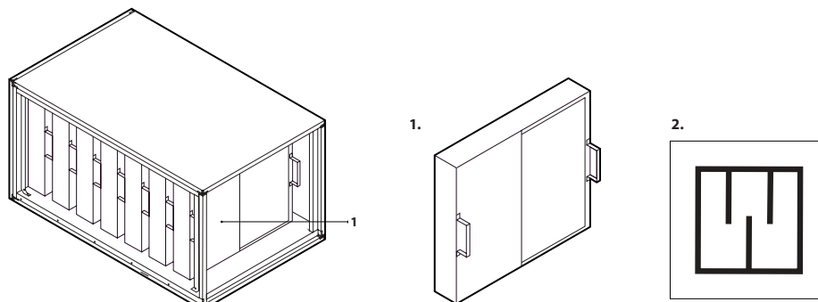
Fig. 8. Sectie Geluidsonderdrukking 1 – verwijderbare geluidsabsorberende wanden, 2 – etiket geluiddempersectie
