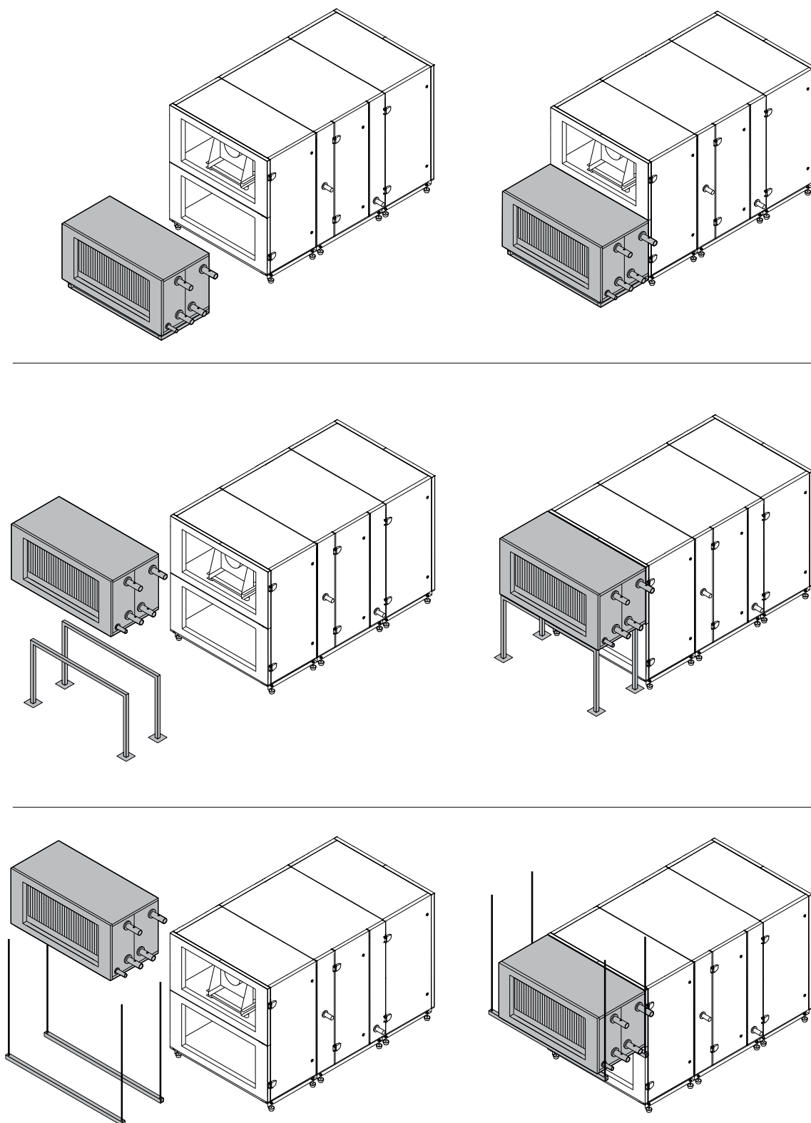
Fig. 17. Voorbeelden voor de installatie van verwarmings-/koelersecties
