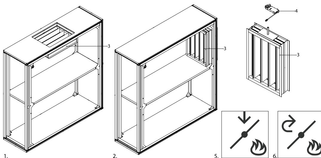
Fig. 9. Rookafvoersectie 1 – rookafvoersectie met klep aan de bovenkant, 2 – rookafvoersectie met klep aan de achterkant, 3 – rookomloopklep, 4 – klepaandrijving, 5 – sectielabel wanneer de klep zich aan de bovenkant bevindt, 6 – sectielabel wanneer de klep aan de achterkant zit
