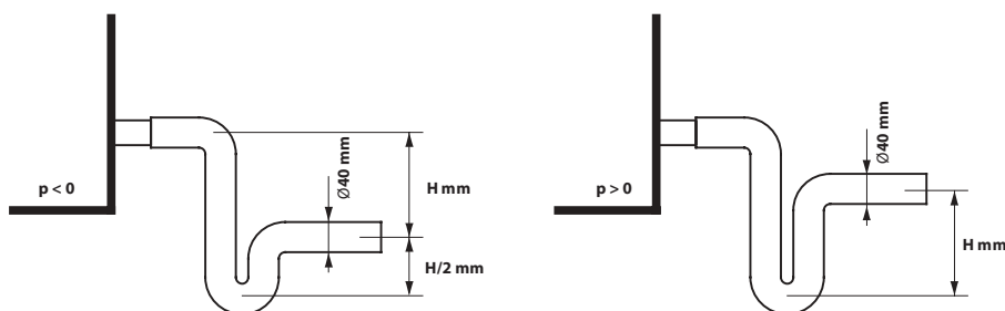
Fig. 21. Installatie van een sifon zonder eenrichtingsklep
