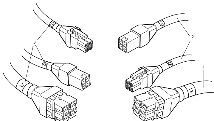
Fig. 39. Kabelverbindingen tussen secties 1 – voedingskabel, 2 – communicatiekabels tussen printplaten 3 – labels met aansluitingsnummers
