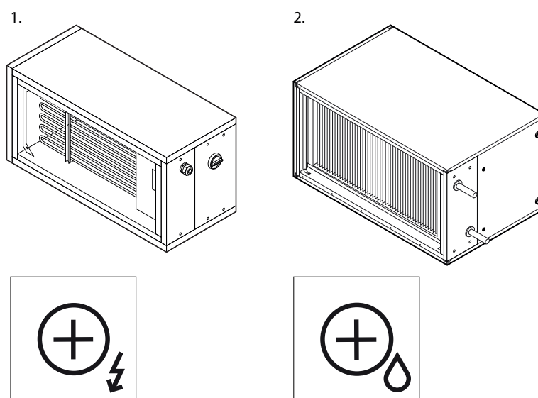
Fig. 6. Verwarmingssectie
