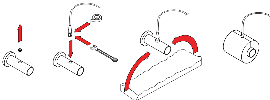
Fig. 20. Installatie van een retourwatertemperatuursensor met schroefdraad 3
