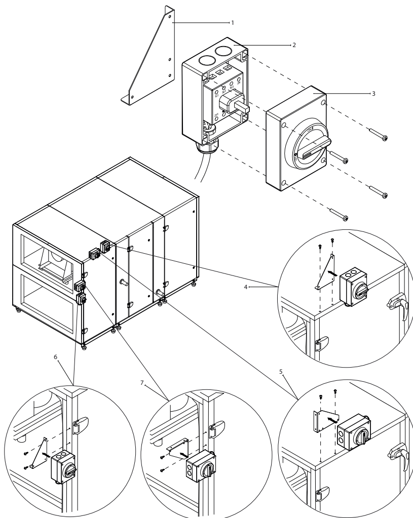
Fig. 28. Hoofdstroomonderbreker en montagevoorbeelden
