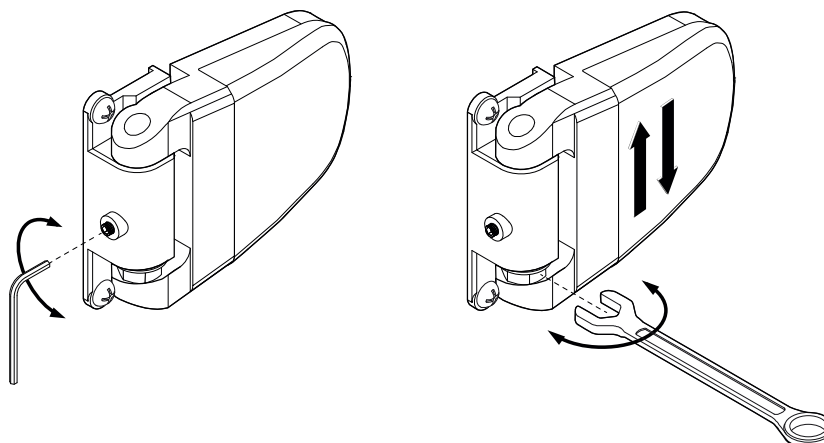
Fig. 14. Aanpassen van de scharnieren
