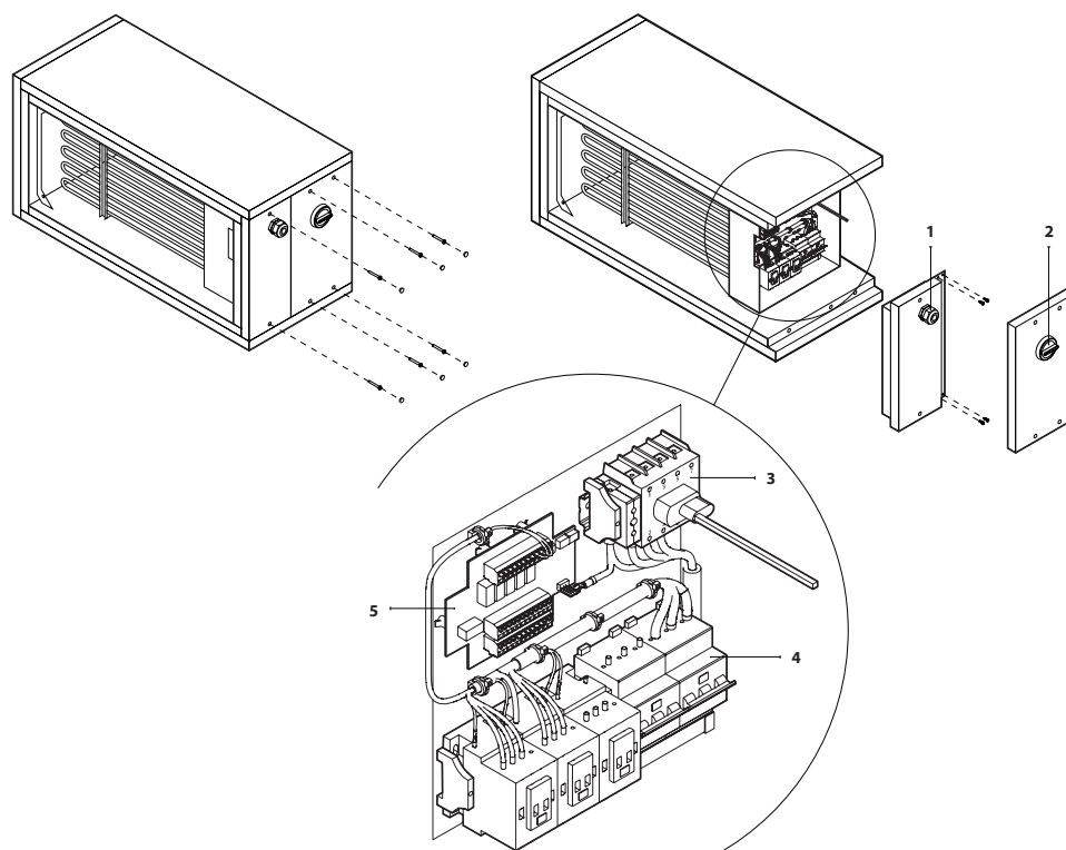
Fig. 29. Hoofdstroomonderbreker in een elektrisch verwarmingssectie 1 – kabeldoorvoertule, 2 – hendel hoofdstroomonderbreker, 3 – hoofdstroomonderbreker, 4 – automatische schakelaar, 5 – bedieningspaneel elektronische verwarmers
