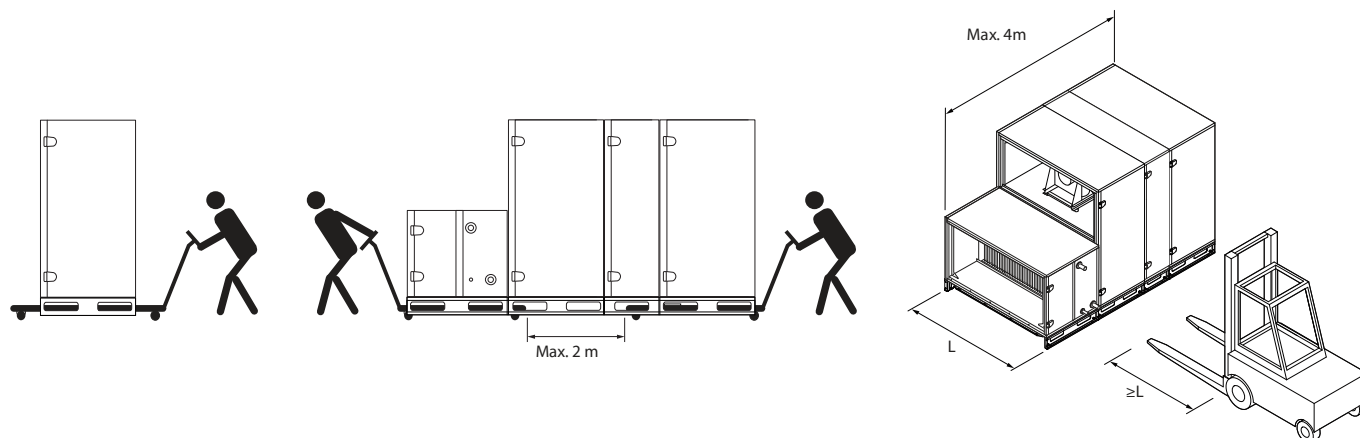
Fig. 10. Kastvervoer met behulp van een vorkheftruck of een trolley
