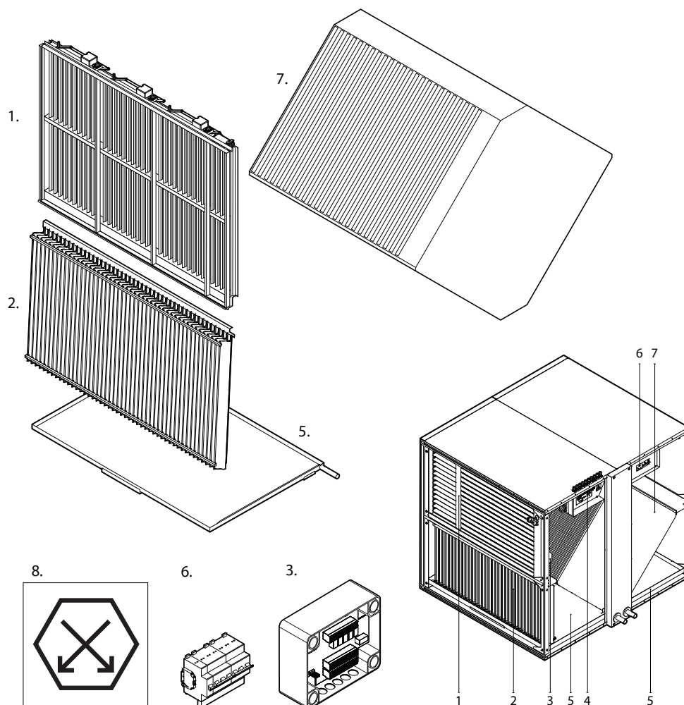
Fig. 2. Sectie Tegenstroomwarmtewisselaar (CF)
