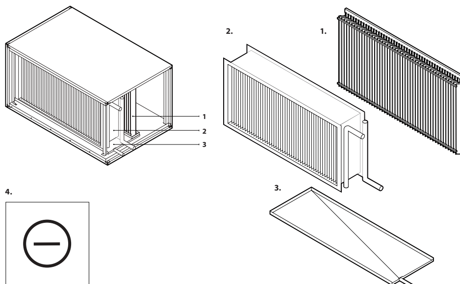
Fig. 5. Koelersectie 1 – druppelvanger, 2 – spoel voor water/koelmiddel 3 – condensbak, 4 – etiket koelersectie
