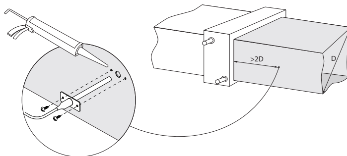
Fig. 36. Installatie van een toevoerluchttemperatuursensor
