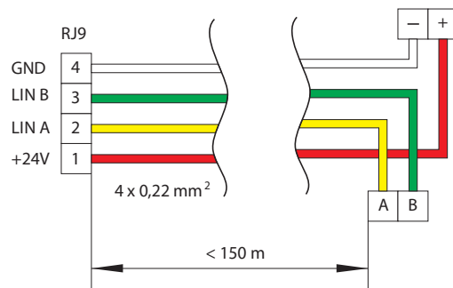
Fig. 37. Bedieningspaneel bedradingsschema
