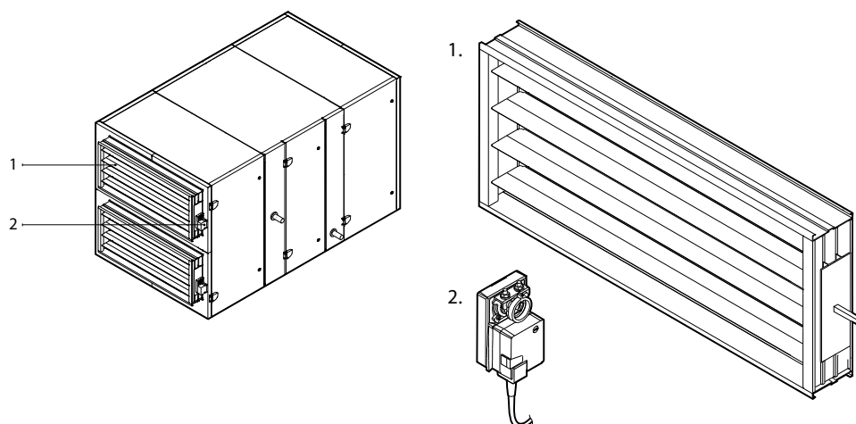
Fig. 7. Luchtafsluitende kleppen
