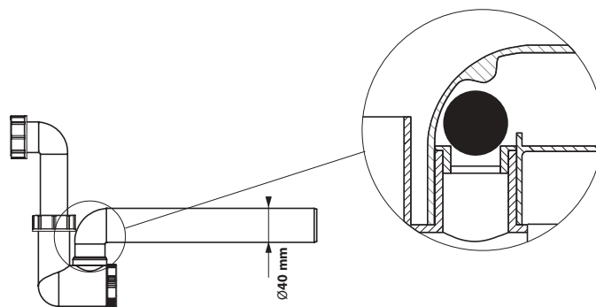
Fig. 22. Voorbeeld van een sifon met een eenrichtingsklep
