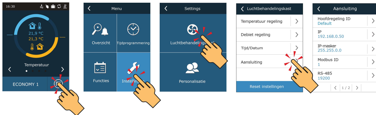
Fig. 41. Het bekijken en wijzigen van het IP-adres met een bedieningspaneel
