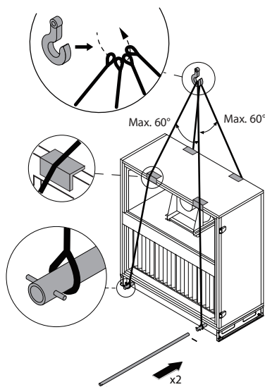
Fig. 11. Hijsen van afzonderlijke secties 1
