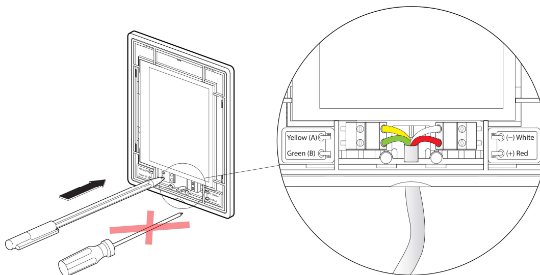
Fig. 38. Bedrading bedieningspaneel
