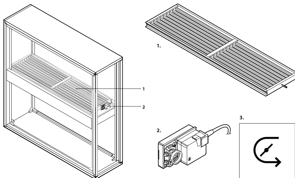
Fig. 4. Recirculatiesectie 1 – luchtmengklep, 2 – klepaandrijving, 3 – etiket recirculatiesectie
