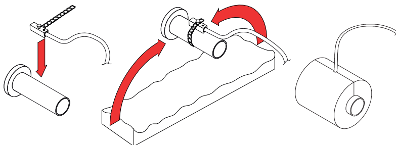
Fig. 19. Installatie van een aan de oppervlakte gemonteerde temperatuursensor voor het retourwater 2
