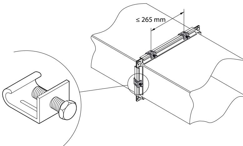
Fig. 25. Voorbeeld van kanaalaansluiting met universele klemverbanden
