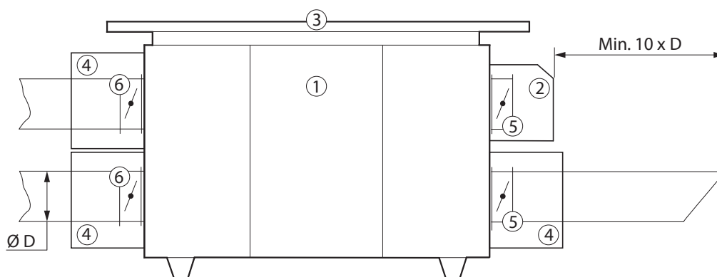
Afb. 26. Accessoires voor kasten die buiten worden geïnstalleerd
