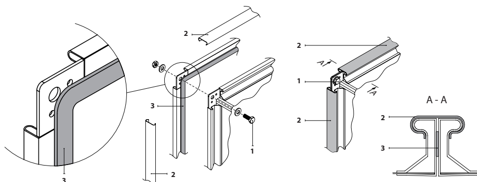
Fig. 24. Voorbeeld voor het bevestigen en afdichten van een flenskanaalverbinding 1 – schroef, 2 – C-profiel voor het aansluiten van flenzen, 3 – zelfklevende pakking
