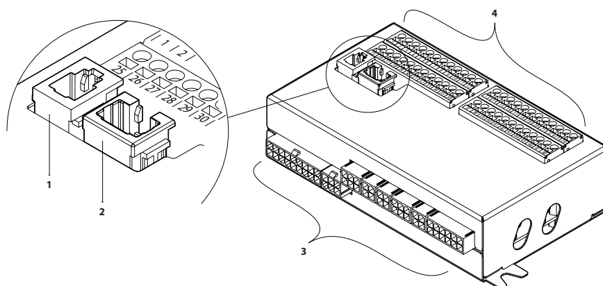
Fig. 31. Hoofdpaneel van het C5-bedieningspaneel
