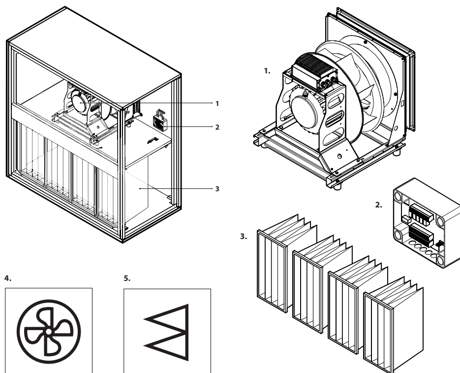
Fig. 1. Filterventilatorsectie
