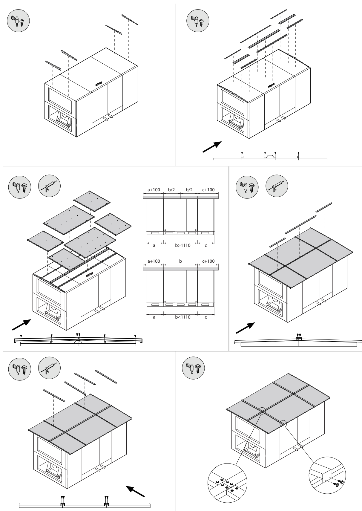
Fig. 27. Installatie van een afzonderlijk besteld beschermend dak 1
