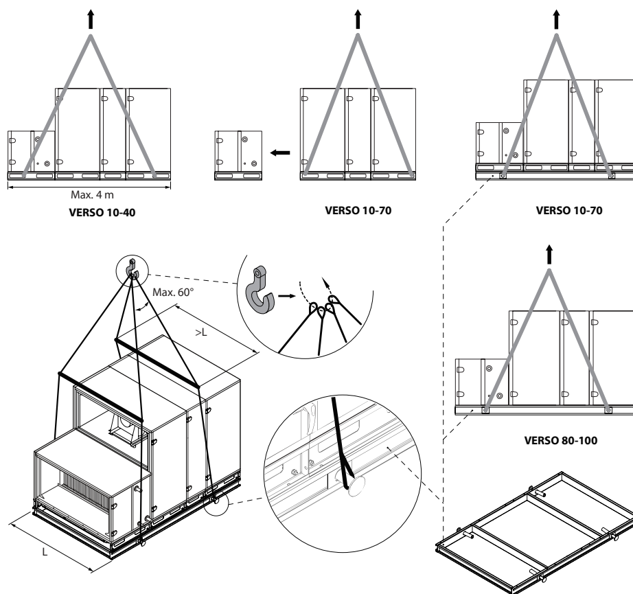
Fig. 12. LBK volledig gemonteerd op een versterkt montageframe tillen 1
