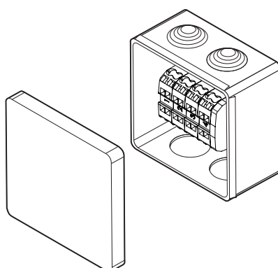
Fig. 40. Aftakdoos PD1
