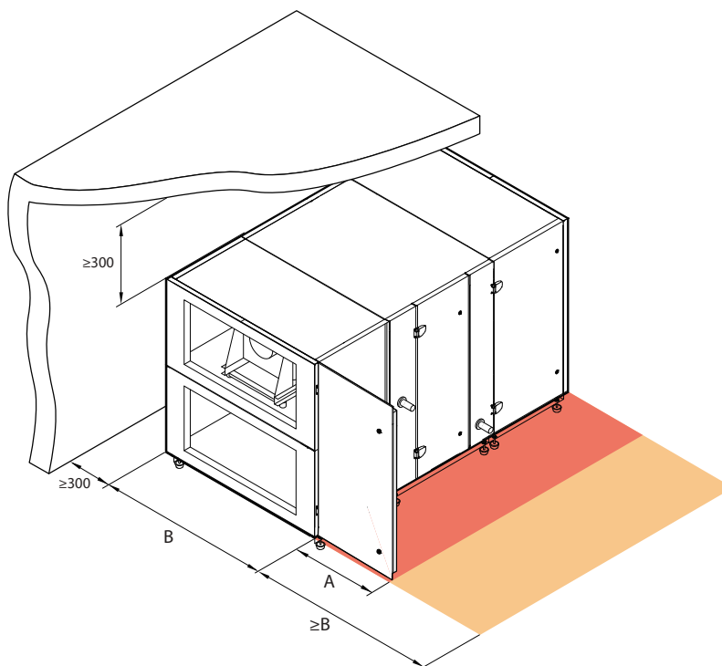
Fig. 15. Kastinspectiegebied
