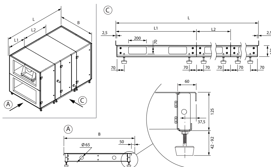
Fig. 13. Inbouwframe met verstelbare poten
