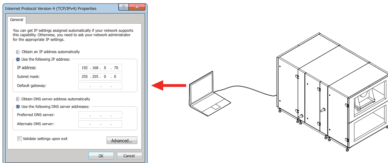
Fig. 42. Computernetwerkinstellingen voor directe aansluiting op de kast
