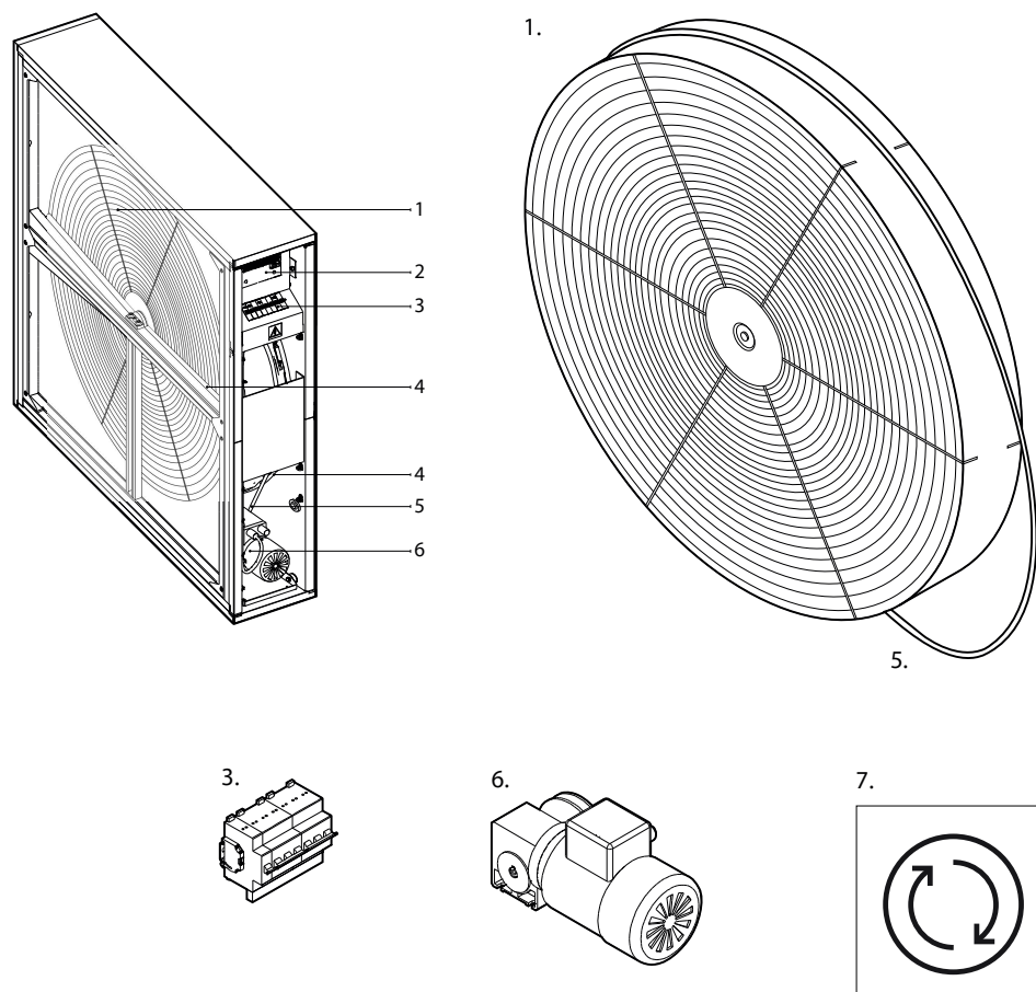
Fig. 3. Sectie Roterende Recuperator 1 – rotorwiel, 2 – automatiseringskast, 3 – automatische schakelaar, 4 – rotorwielborstelafdichtingen, 5 – rotorriem, 6 – rotorreductiemotor, 7 – etiket rotorsectie
