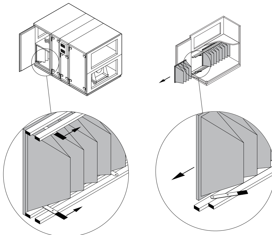
Fig. 4 Filterklemminrichting
