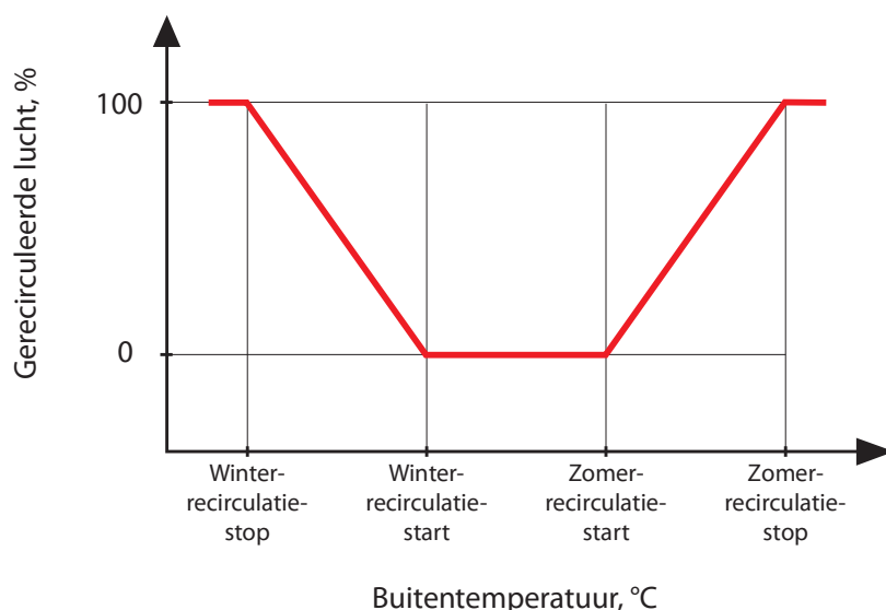
Fig. 3 REC-functiebediening
