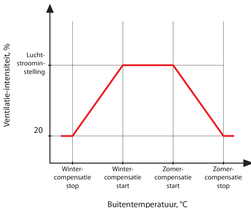
Fig. 2 OCV-functiebediening
