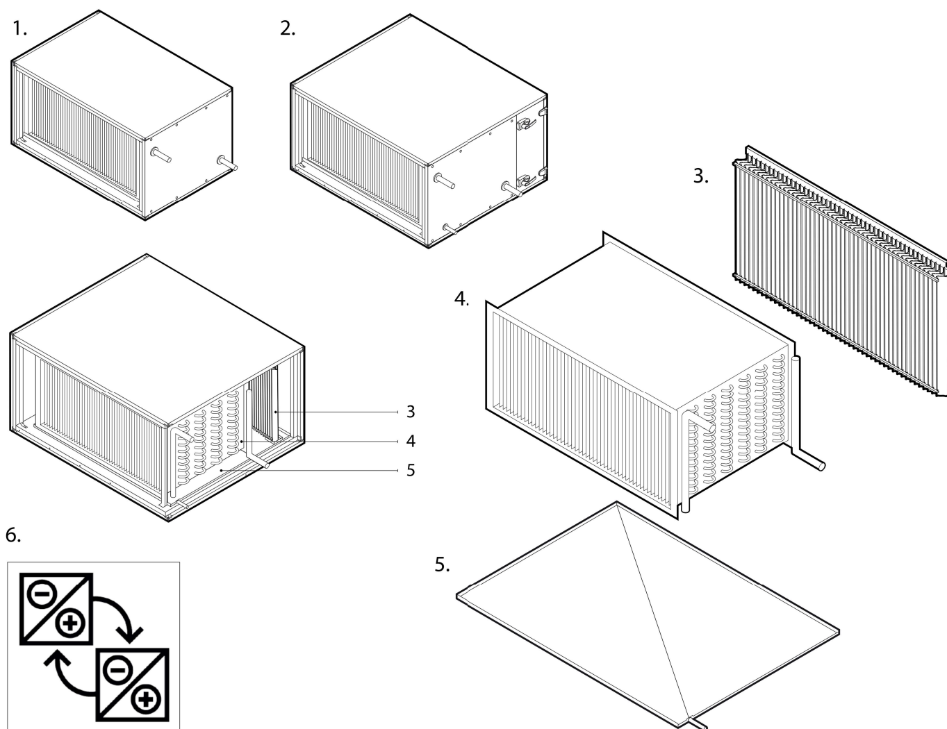
Fig. 4. Secties van vloeistofgekoppelde warmtewisselaar
