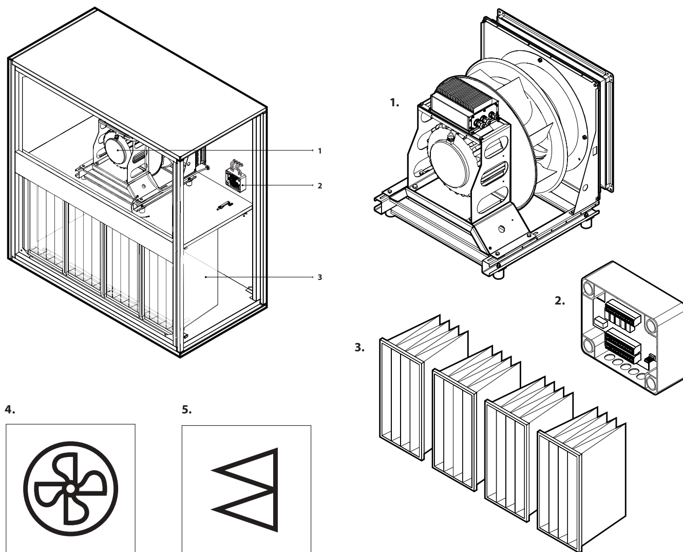
Fig. 1. Filtrventilatorsectie
