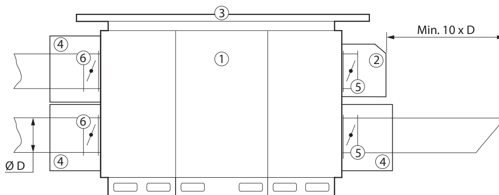
Afb. 33. Accessoires voor kasten die buiten worden geïnstalleerd
