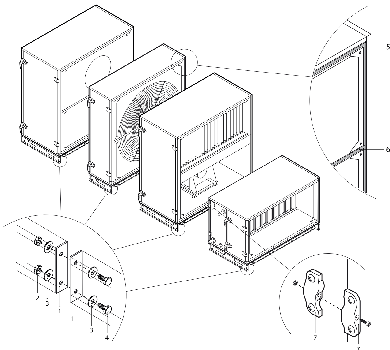
Fig. 21. Externe aansluiting en afdichting van secties
