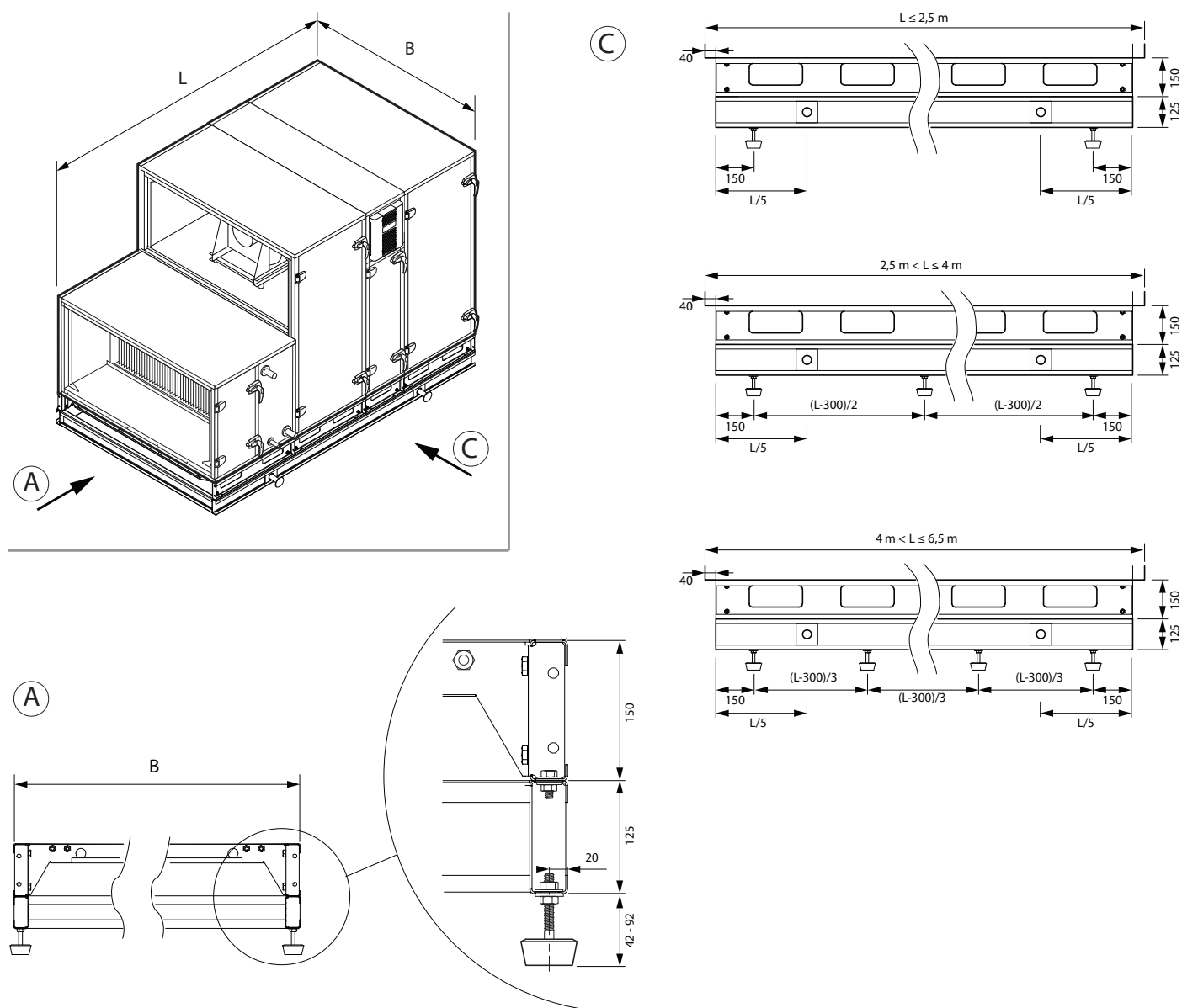
Fig. 16. Afmetingen van het versterkt montageframe
