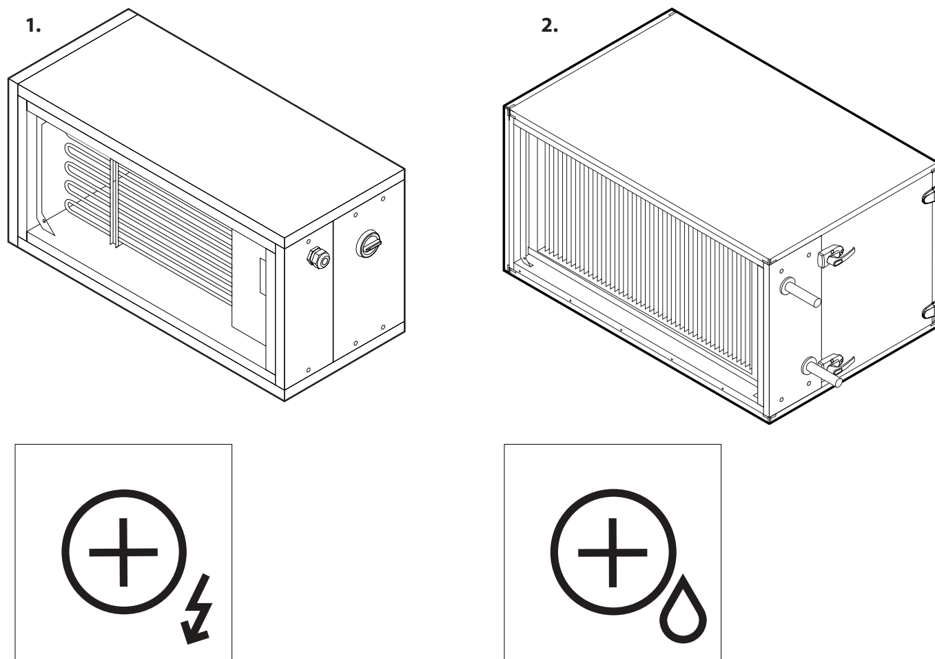
Fig. 7. Verwarmingssectie
