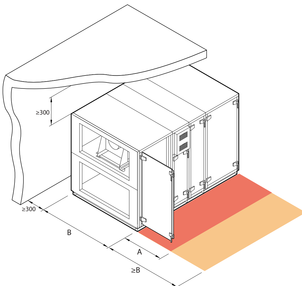
Fig. 18. Kastinspectiegebied
