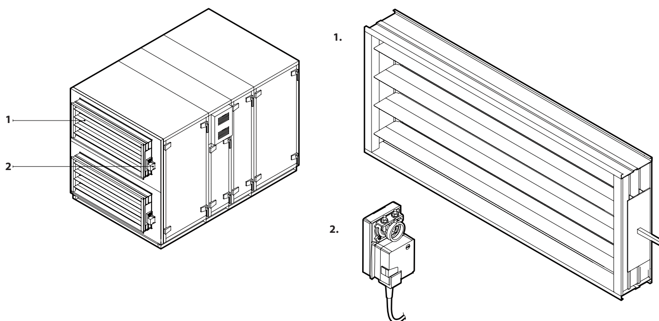
Fig. 8. Luchtafsluitende kleppen 1 – luchtklep, 2 – elektrische klepaandrijving
