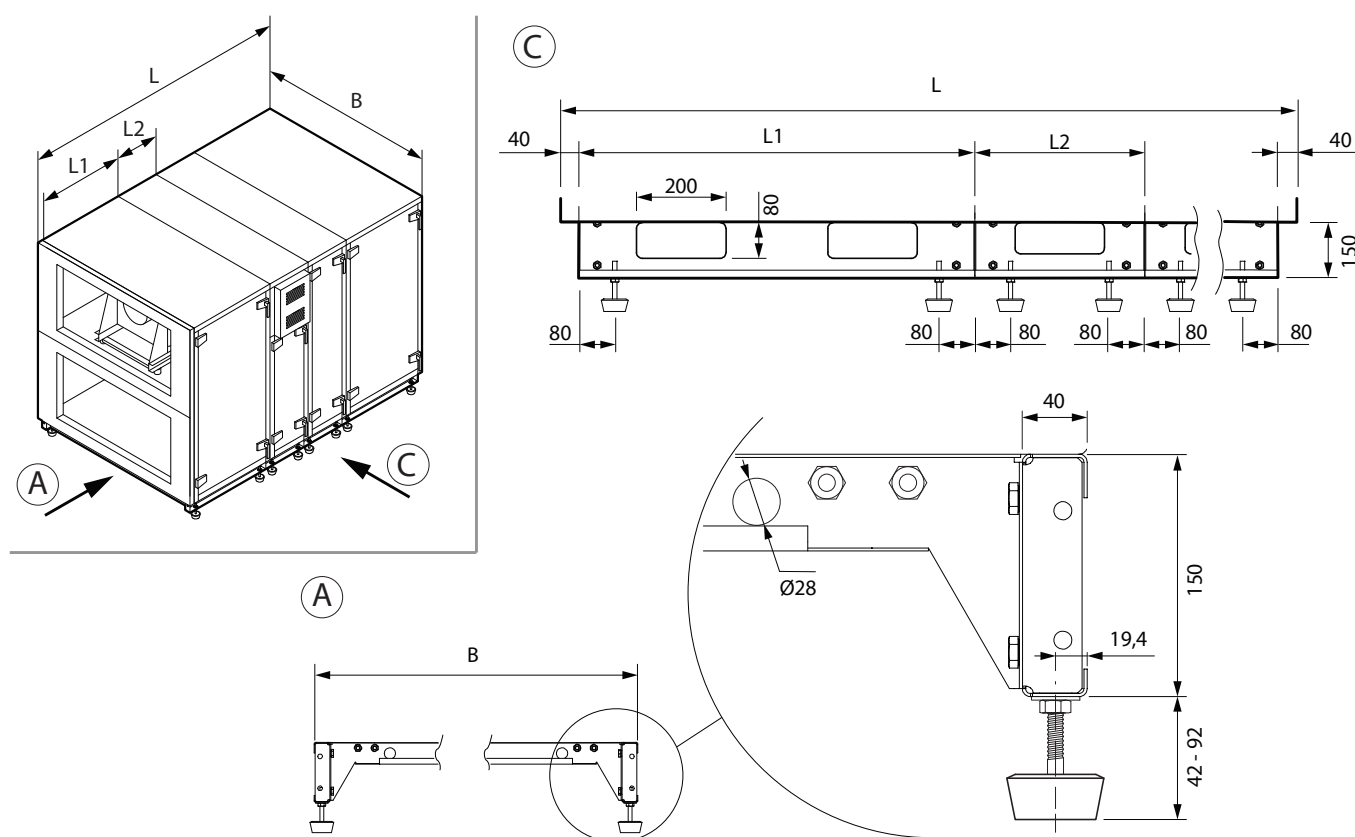
Fig. 17. Inbouwframe met verstelbare poten
