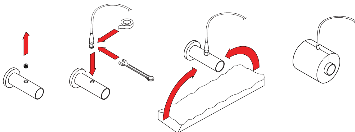
Fig. 27. Installatie van een retourwatertemperatuursensor met schroefdraad 1
