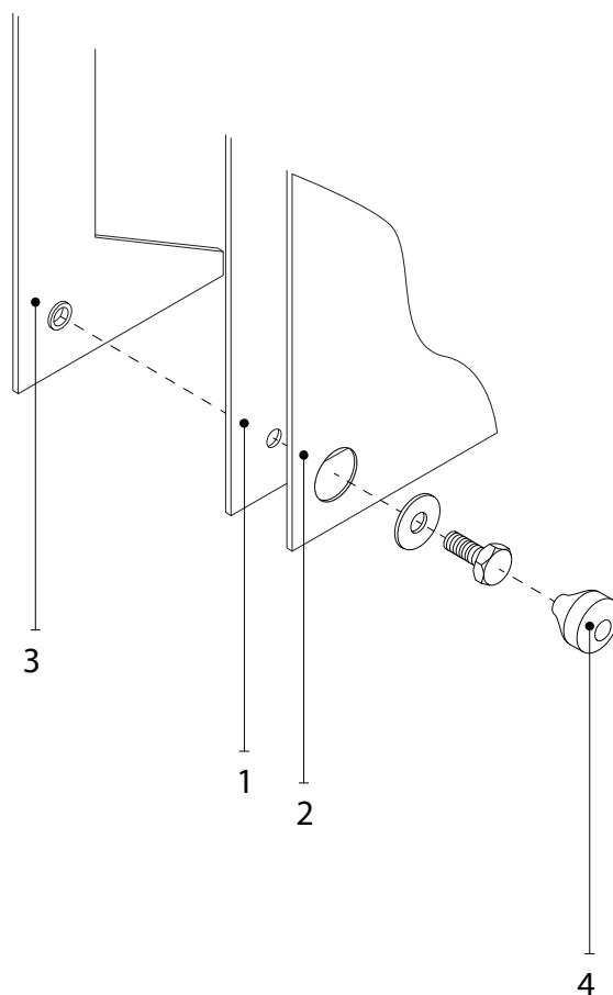
Fig. 23. Interne aansluiting in een ventilatorsectie
