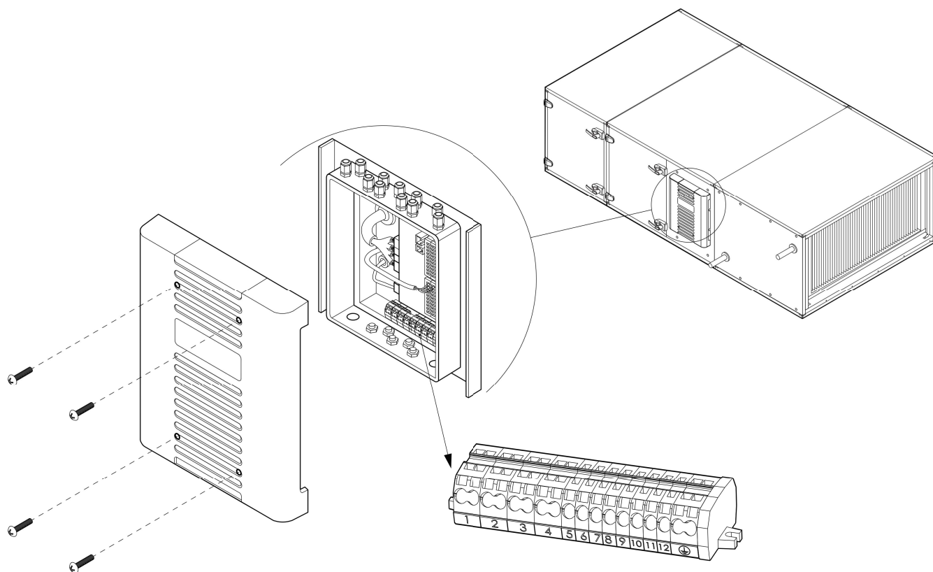
Fig. 46. Aansluitklemmen van VERSO RA luchtbehandelingskasten
