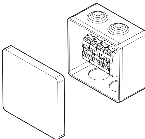
Fig. 51. Aftakdoos PD1
