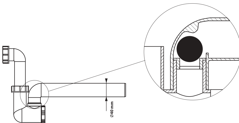
Fig. 29. Voorbeeld van een sifon met een eenrichtingsklep
