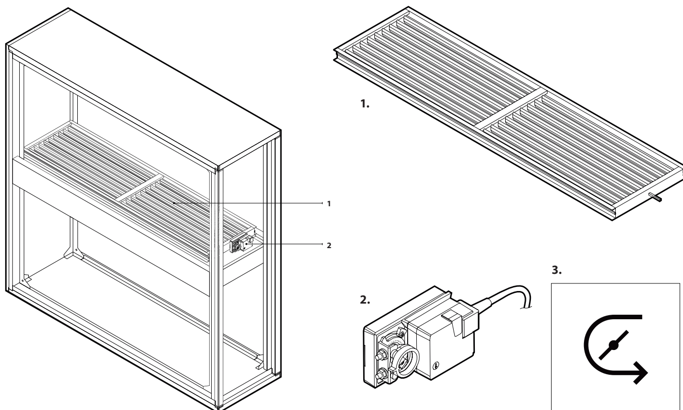
Fig. 5. Recirculatiesectie
