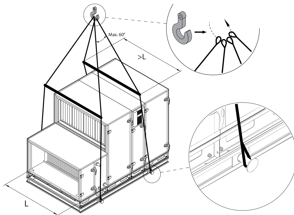
Fig. 15. LBK volledig gemonteerd op een versterkt montageframe tillen 1
