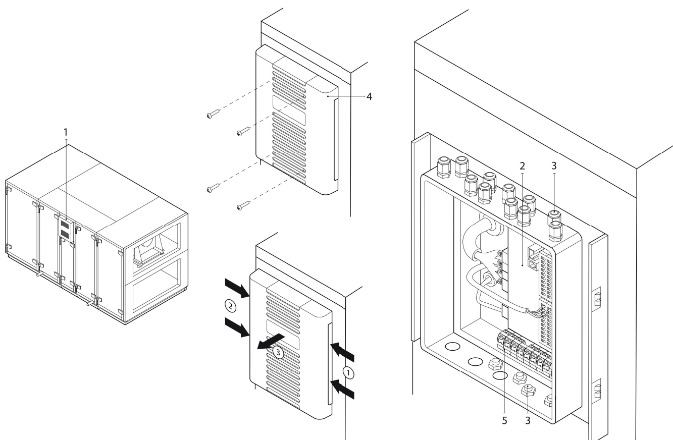
Fig. 37. Automatiseringskast
