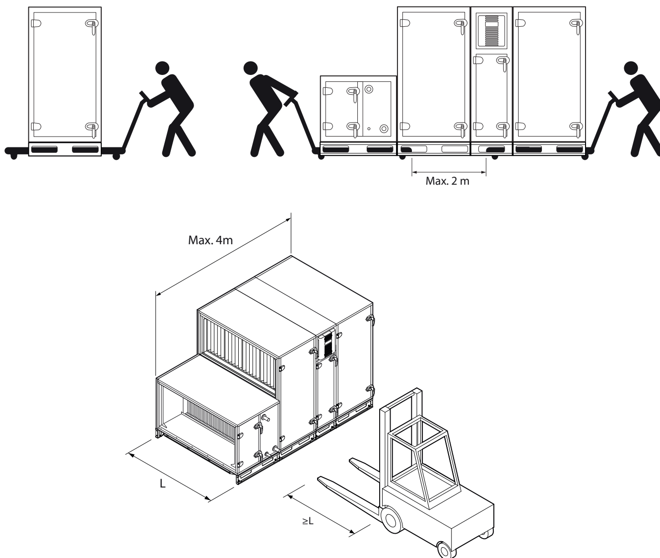
Fig. 13. Kastvervoer met behulp van een vorkheftruck of een trolley
