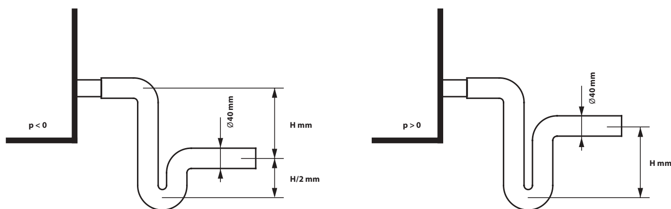
Fig. 28. Installatie van een sifon zonder eenrichtingsklep
