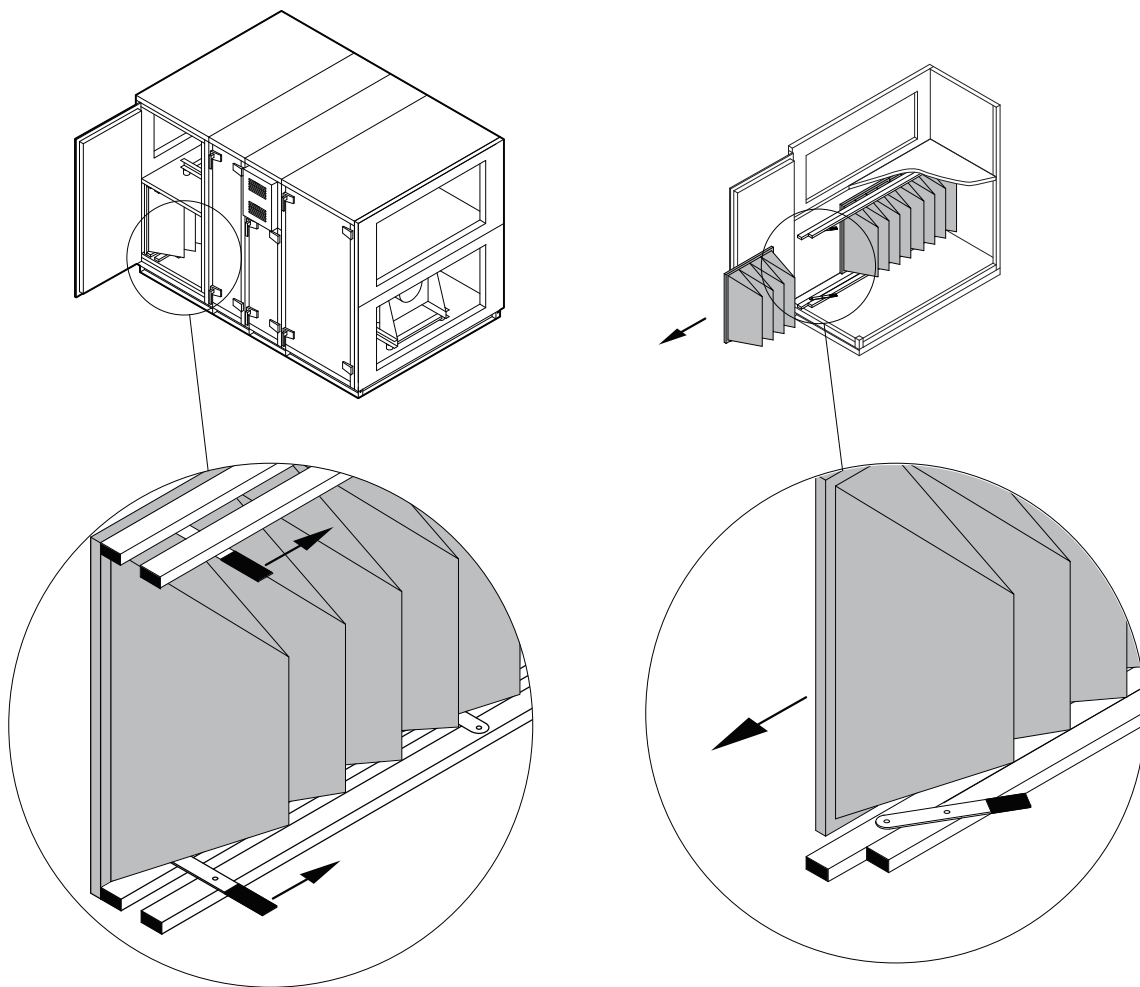
Fig. 55. Filterkleminrichting
