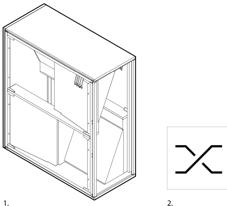
Fig. 12. Luchtstroomwisselingssectie 1 – luchtstroomwisselingssectie, 2 – sectie-etiket
