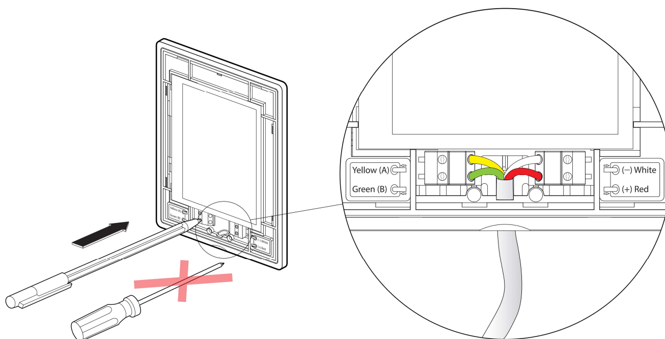
Fig. 49. Bedrading bedieningspaneel
