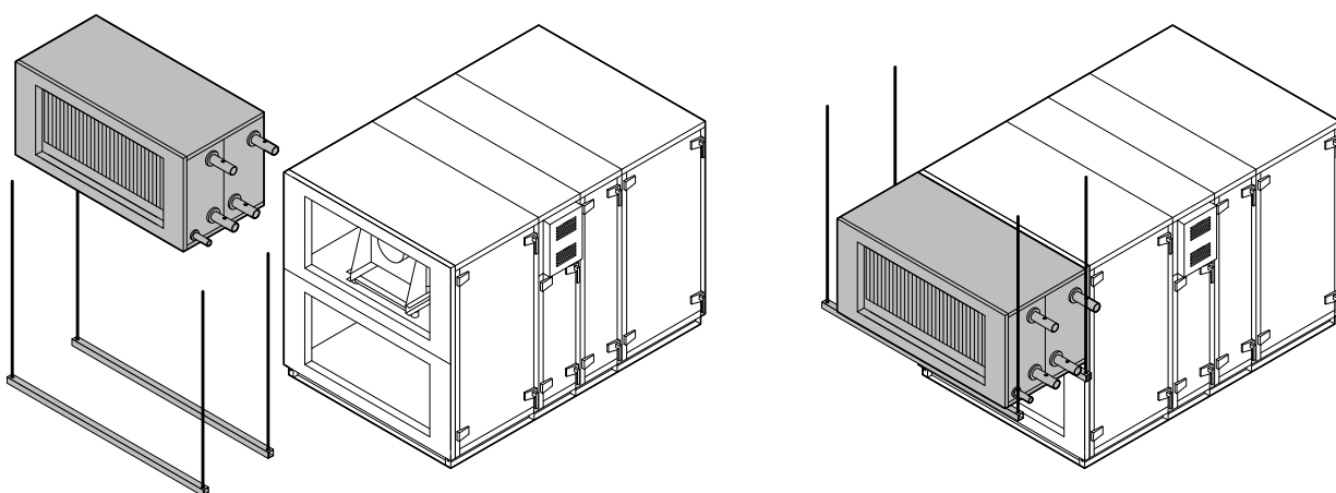
Fig. 24. Voorbeelden voor de installatie van verwarmings-/koelersecties
