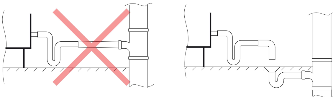
Fig. 30. Aansluiting van de condensatafvoer op de riolering
