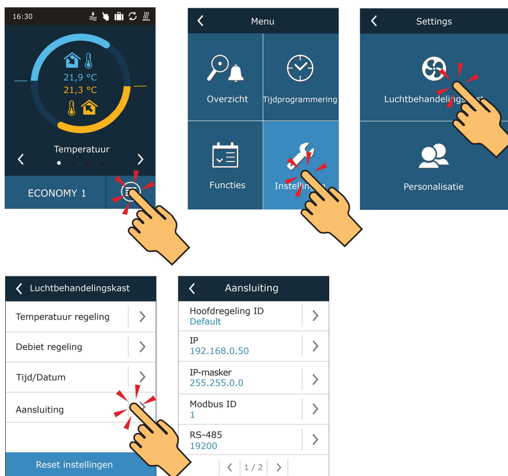
Fig. 52. Het bekijken en wijzigen van het IP-adres met een bedieningspaneel
