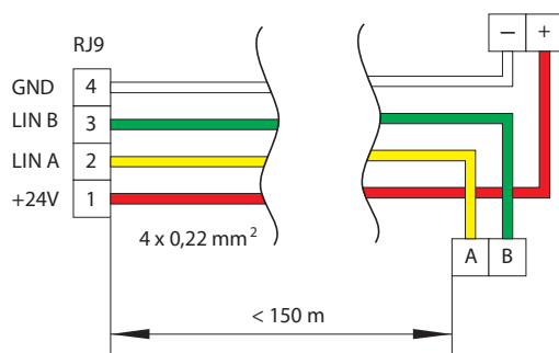
Fig. 48. Bedieningspaneel bedradingsschema
