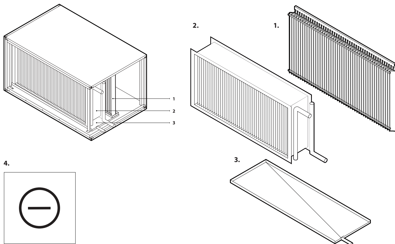
Fig. 6. Koelersectie
