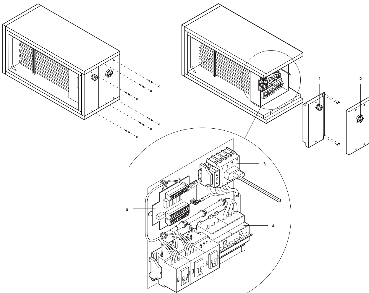
Fig. 36. Hoofdstroomonderbreker in een elektrisch verwarmingssectie
