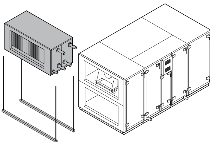
Fig. 24. Voorbeelden voor de installatie van verwarmings-/koelersecties
