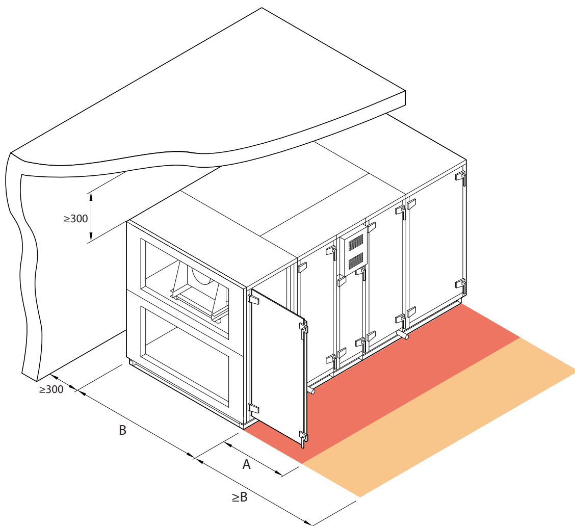
Fig. 18. Kastinspectiegebied
