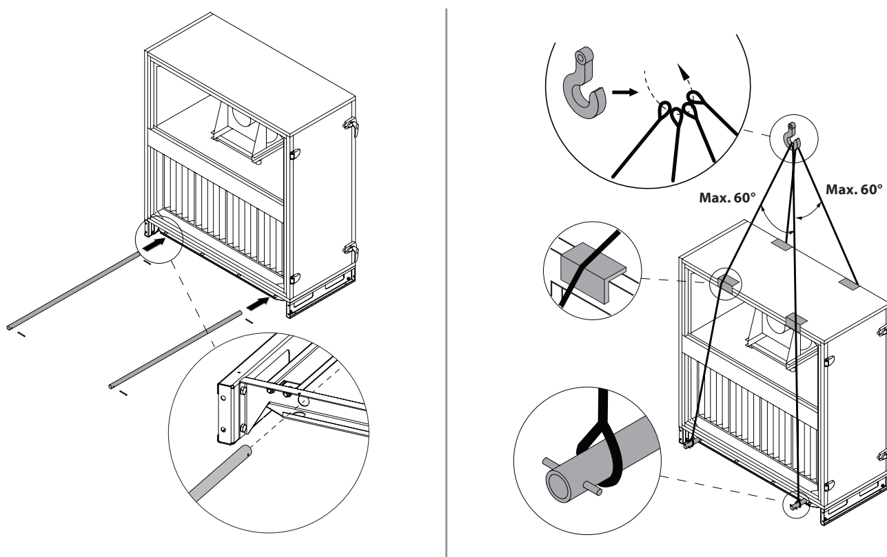
Fig. 14. Hijsen van afzonderlijke secties 1
