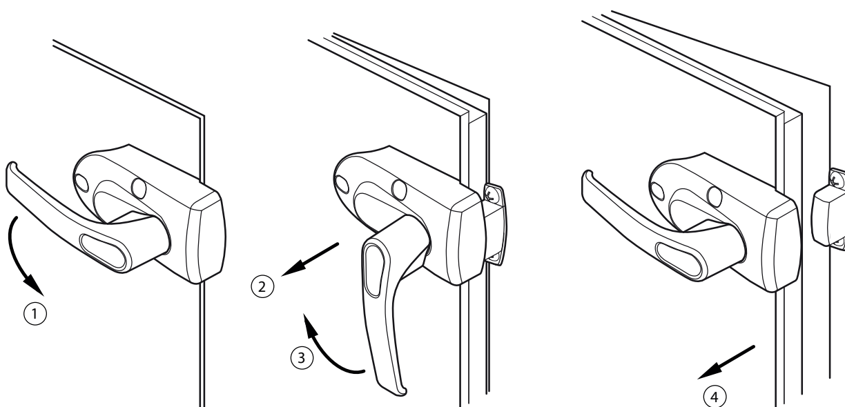
Fig. 19. Het openen van de deur
