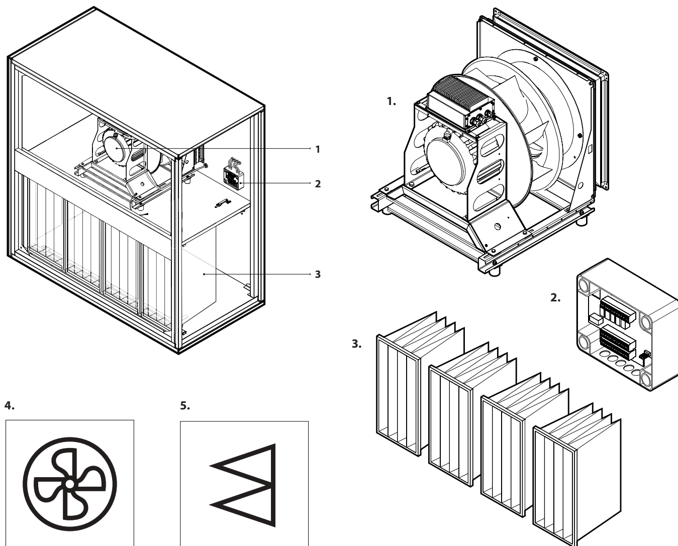
Fig. 1. Filtrventilatorsectie
