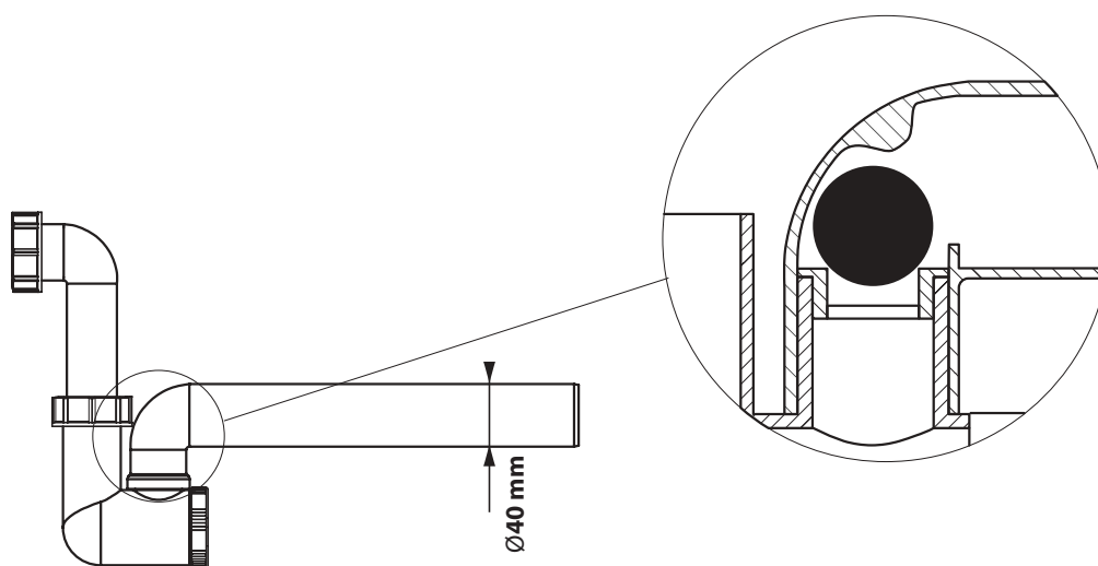
Fig. 29. Voorbeeld van een sifon met een eenrichtingsklep
