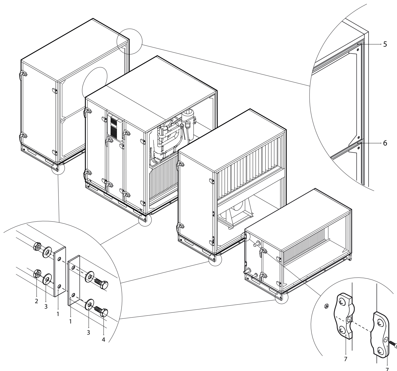
Fig. 21. Externe aansluiting en afdichting van secties
