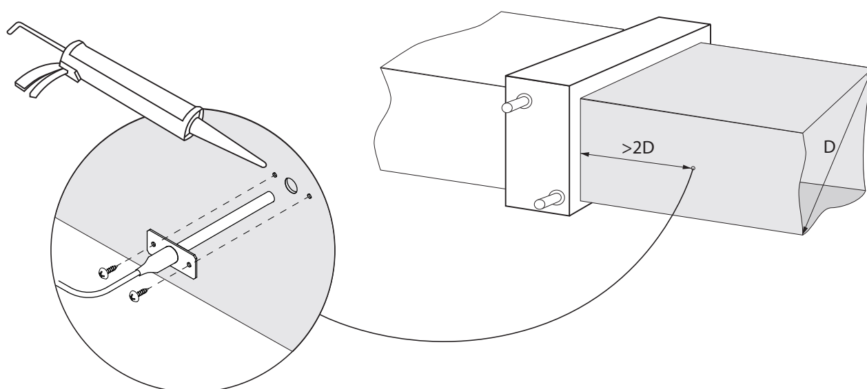
Fig. 43. Installatie van een toevoerluchttemperatuursensor
