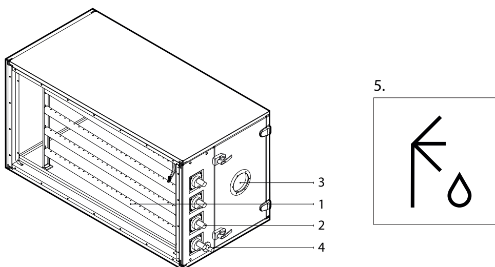
Fig. 11. Luchtbevochtiger
