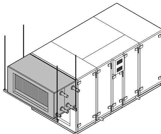
Fig. 24. Voorbeelden voor de installatie van verwarmings-/koelersecties
