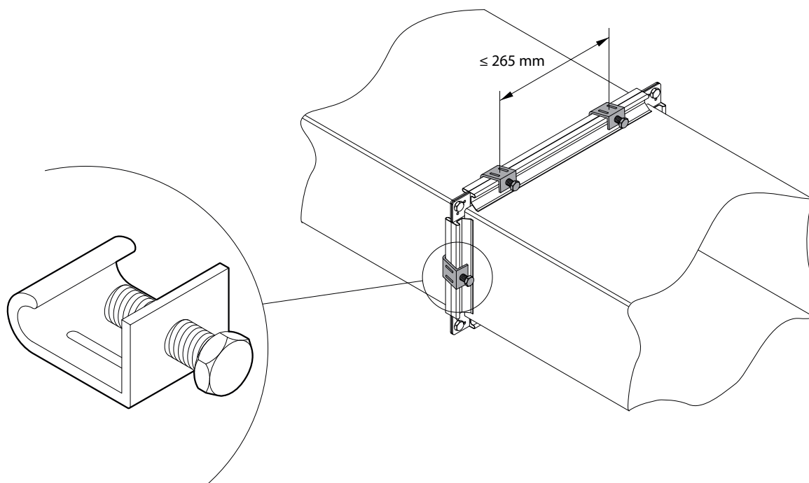
Fig. 32. Voorbeeld van kanaalaansluiting met universele klemverbindingen
