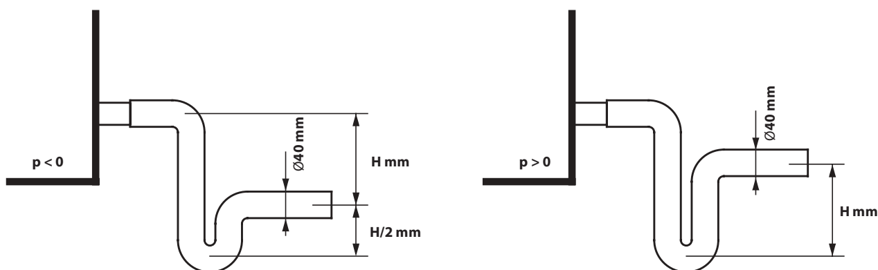
Fig. 28. Installatie van een sifon zonder eenrichtingsklep
