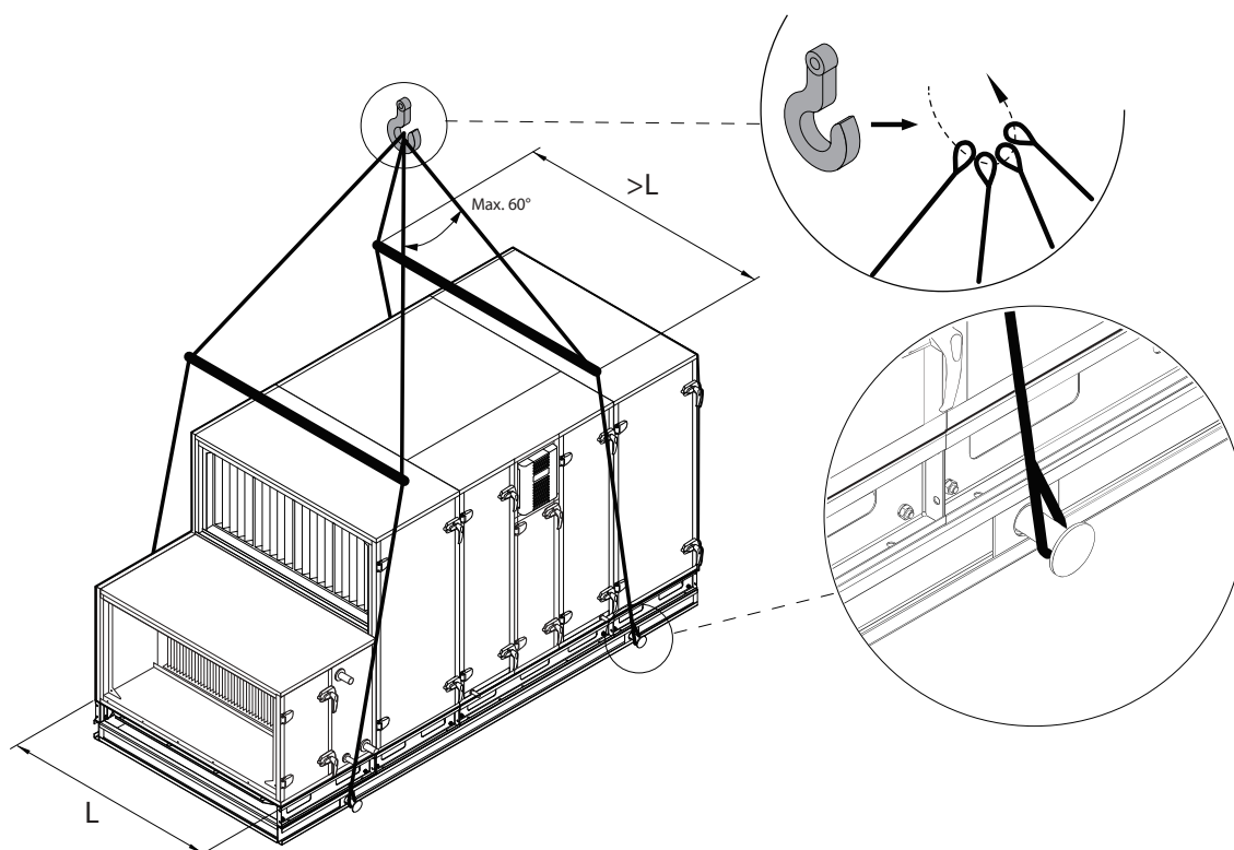
Fig. 15. LBK volledig gemonteerd op een versterkt montageframe tillen 1
