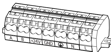
Fig. 44. Extra aansluitklemmenblok
