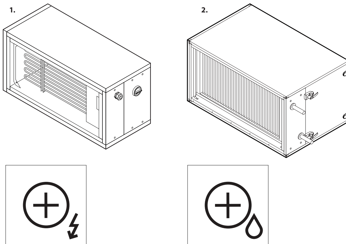
Fig. 8. Verwarmingssectie
