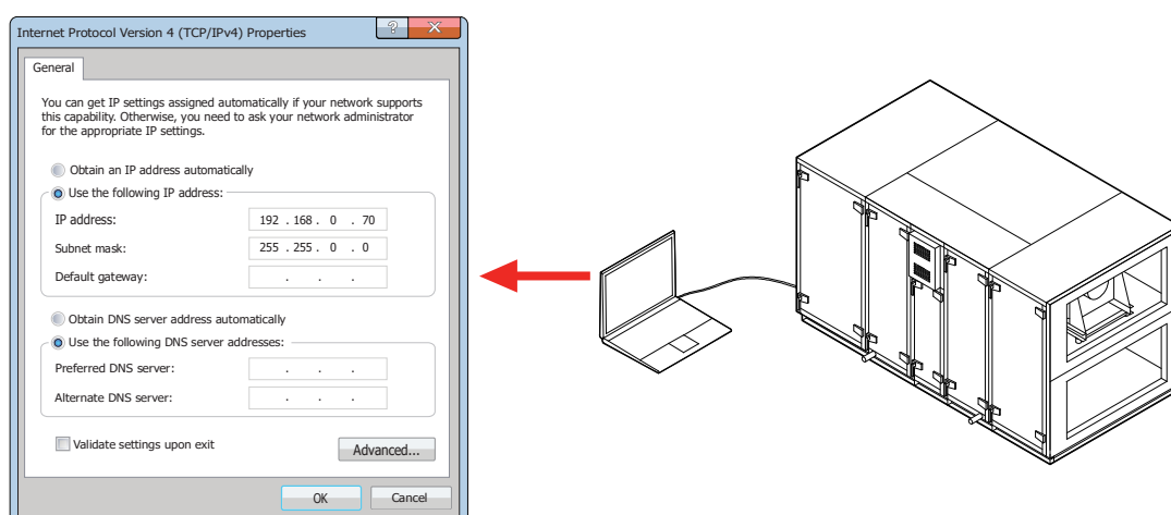
Fig. 51. Computernetwerkinstellingen voor directe aansluiting op de kast
