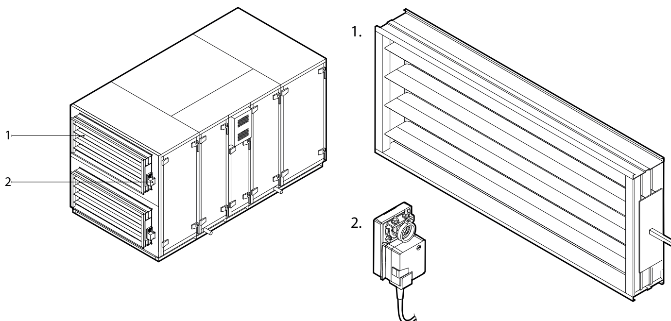
Fig. 9. Luchtafsluitende kleppen 1 – luchtklep, 2 – elektrische klepaandrijving
