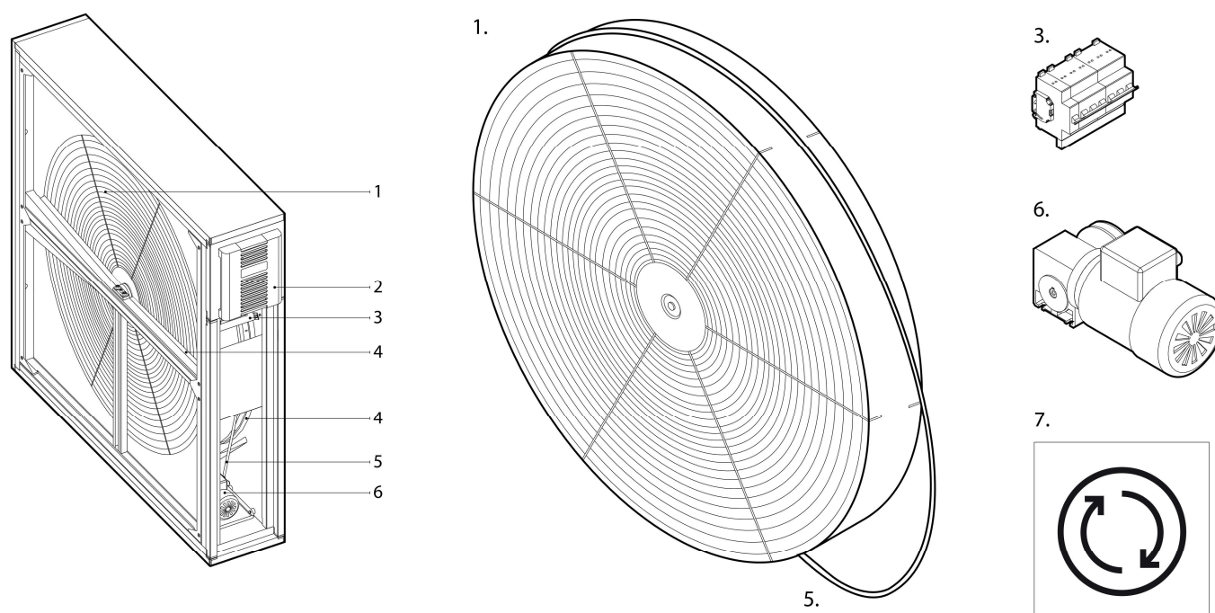
Fig. 3. Sectie Roterende Recuperator
