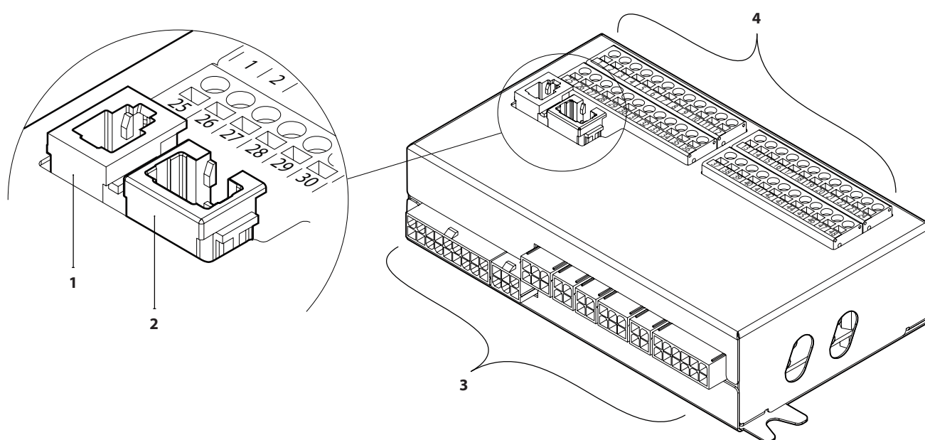
Fig. 38. Hoofdpaneel van het C5-bedieningspaneel
