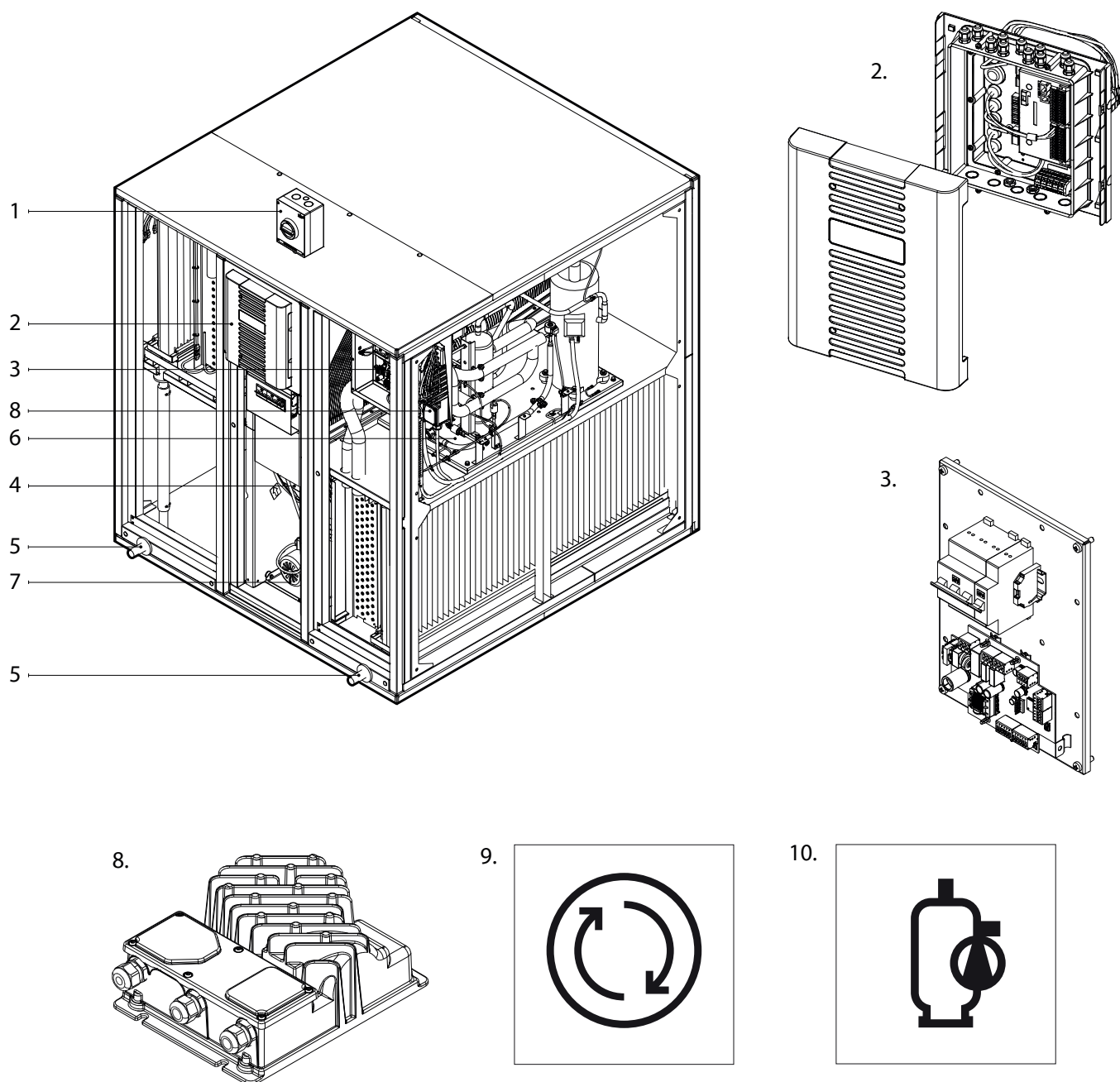
Fig. 2. Warmtepompsectie
