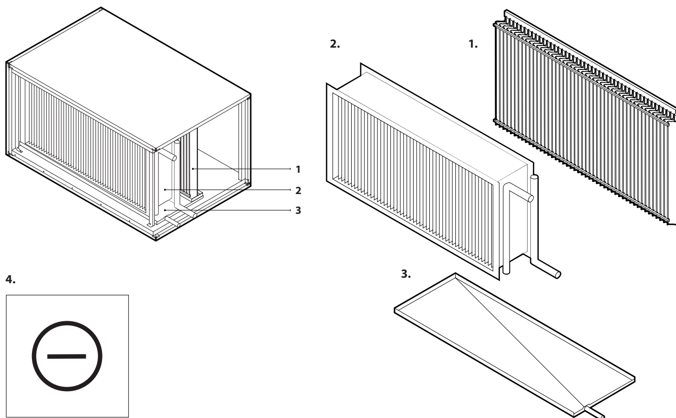
Fig. 7. Koelersectie
