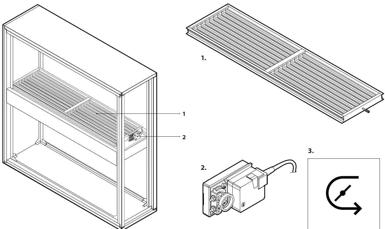
Fig. 6. Recirculatiesectie
