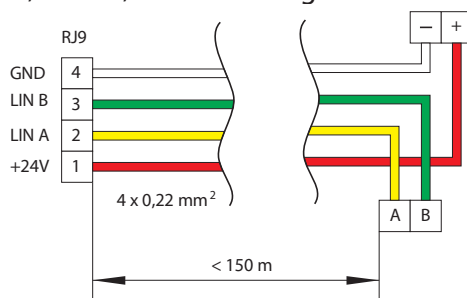
Fig. 46. Bedieningspaneel bedradingsschema
