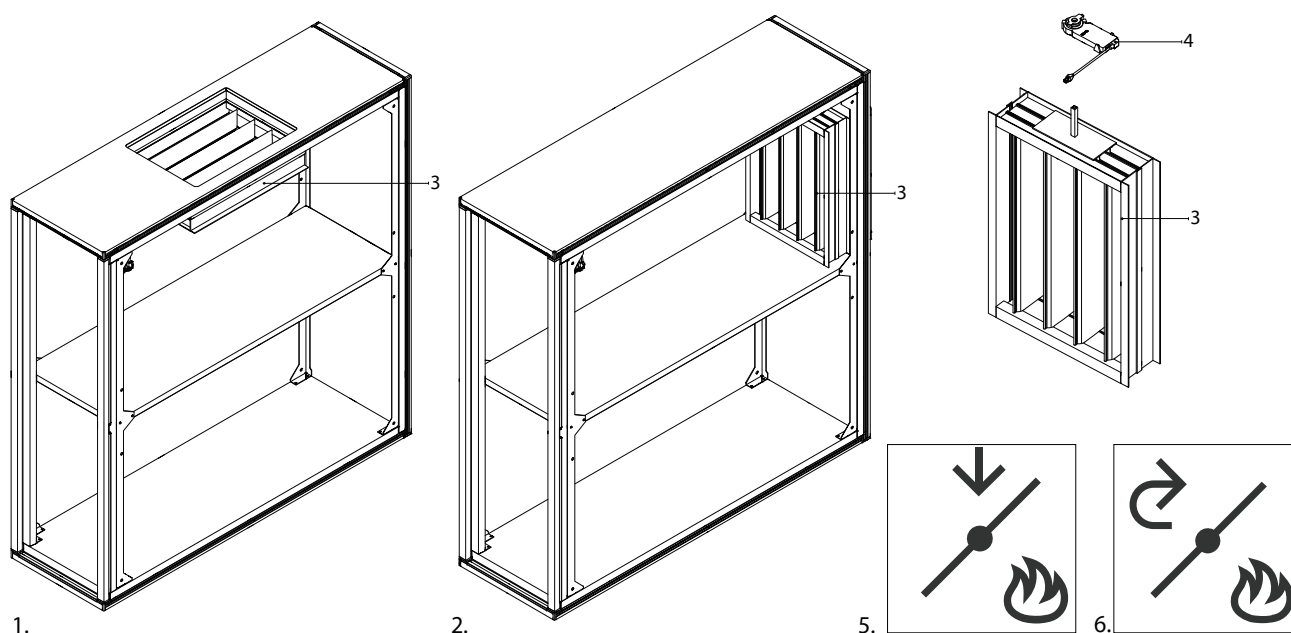
Fig. 12. Rookafvoersectie
