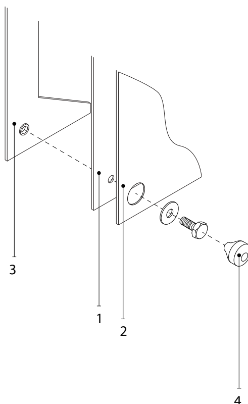
Fig. 23. Interne aansluiting in een ventilatorsectie
