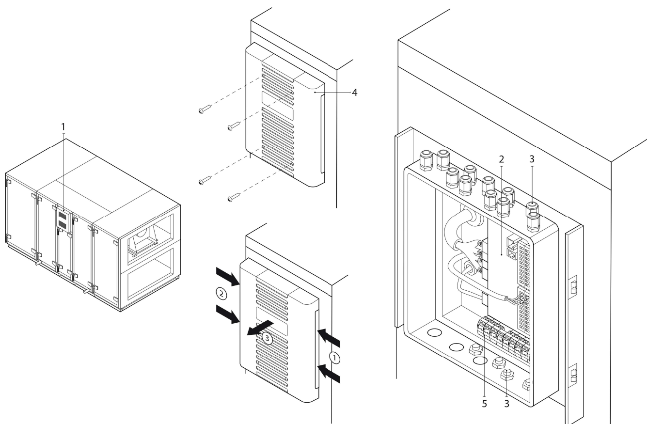
Fig. 37. Automatiseringskast
