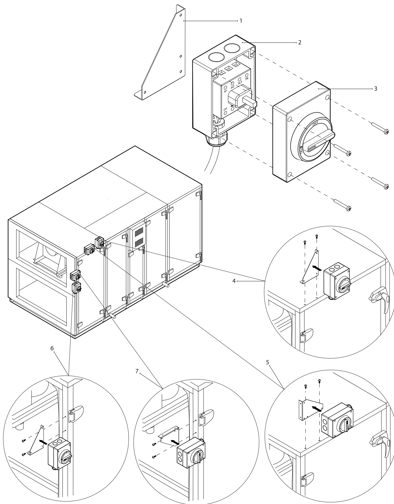
Fig. 35. Hoofdstroomonderbreker en montagevoorbeelden
