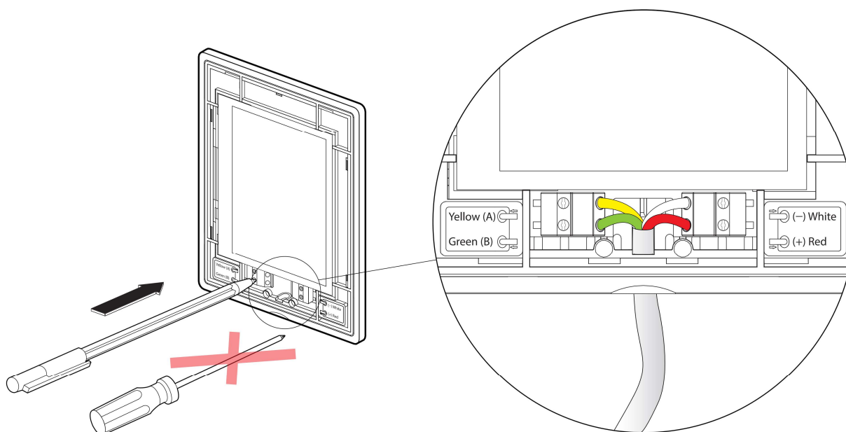
Fig. 47. Bedrading bedieningspaneel
