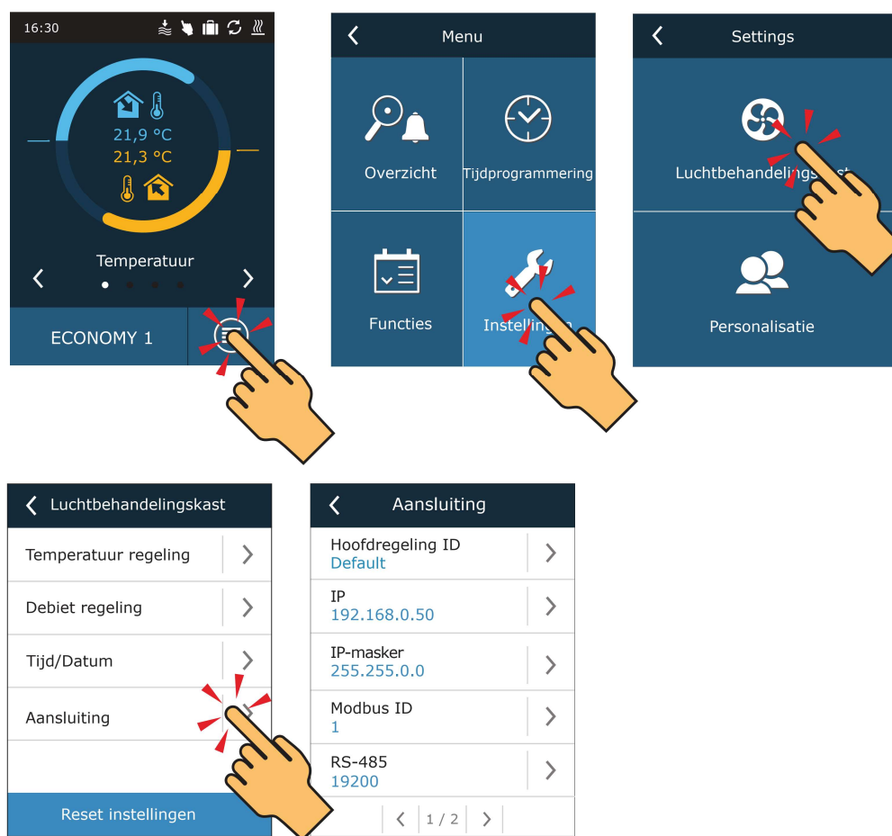
Fig. 50. Het bekijken en wijzigen van het IP-adres met een bedieningspaneel
