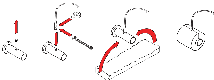
Fig. 27. Installatie van een retourwatertemperatuursensor met schroefdraad 1
