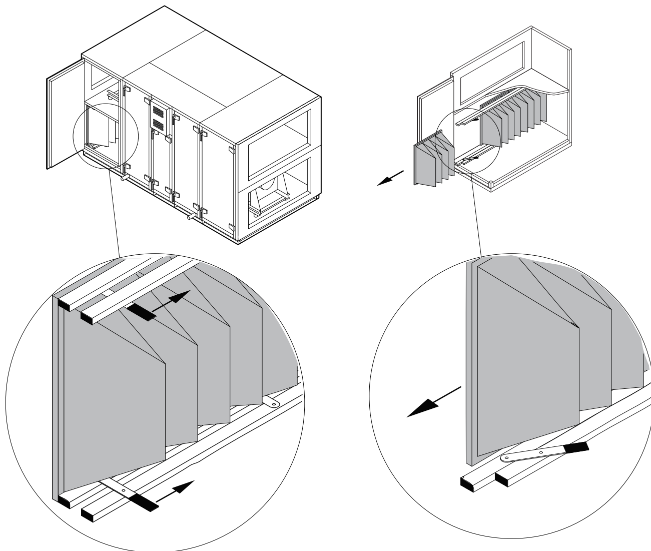
Fig. 3. Filterkleminrichting
